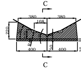
LONGITUDINAL PROFILE
