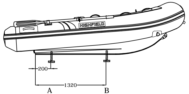
LONGITUDINAL PROFILE
