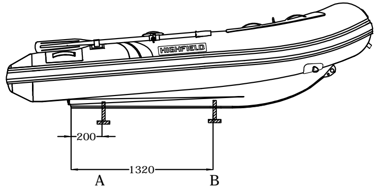
LONGITUDINAL PROFILE
